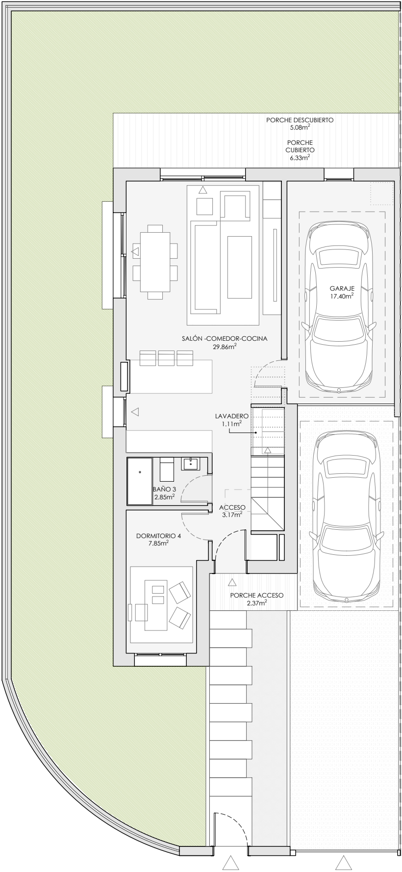
PLANTA BAJA
