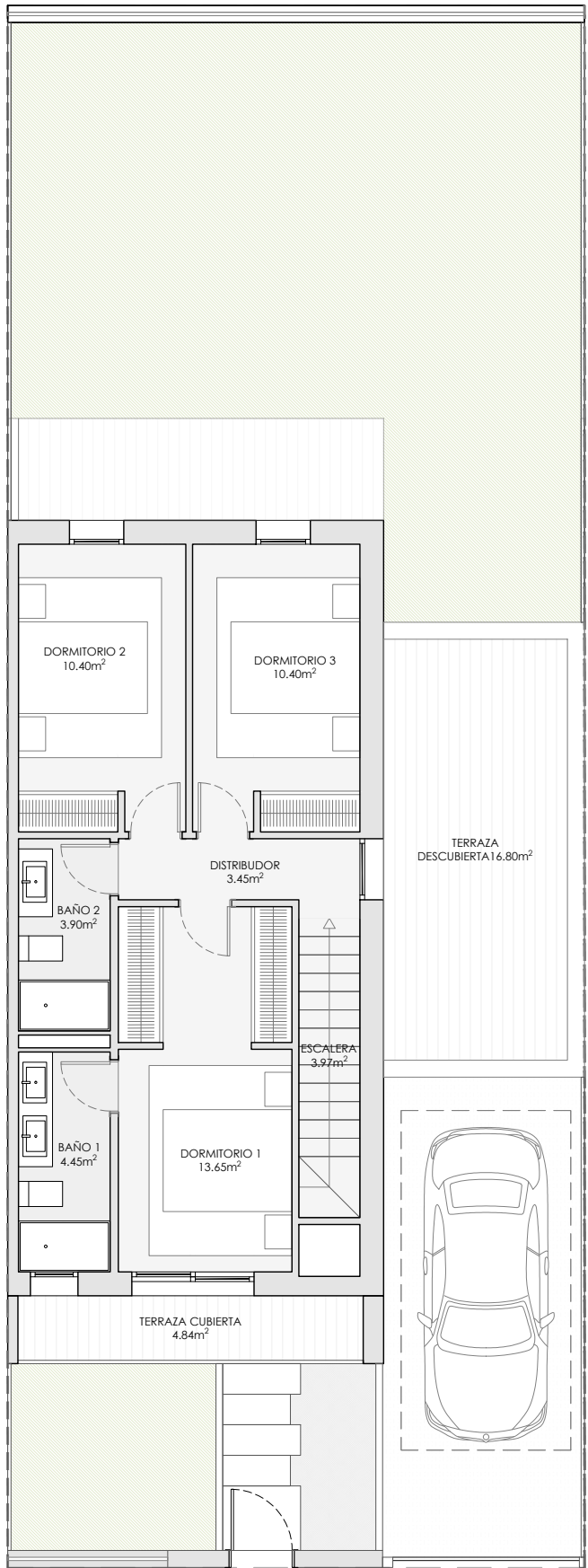
PLANTA PRIMERA
