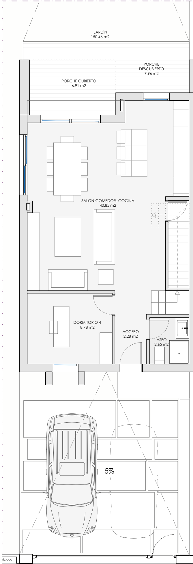
PLANTA BAJA
