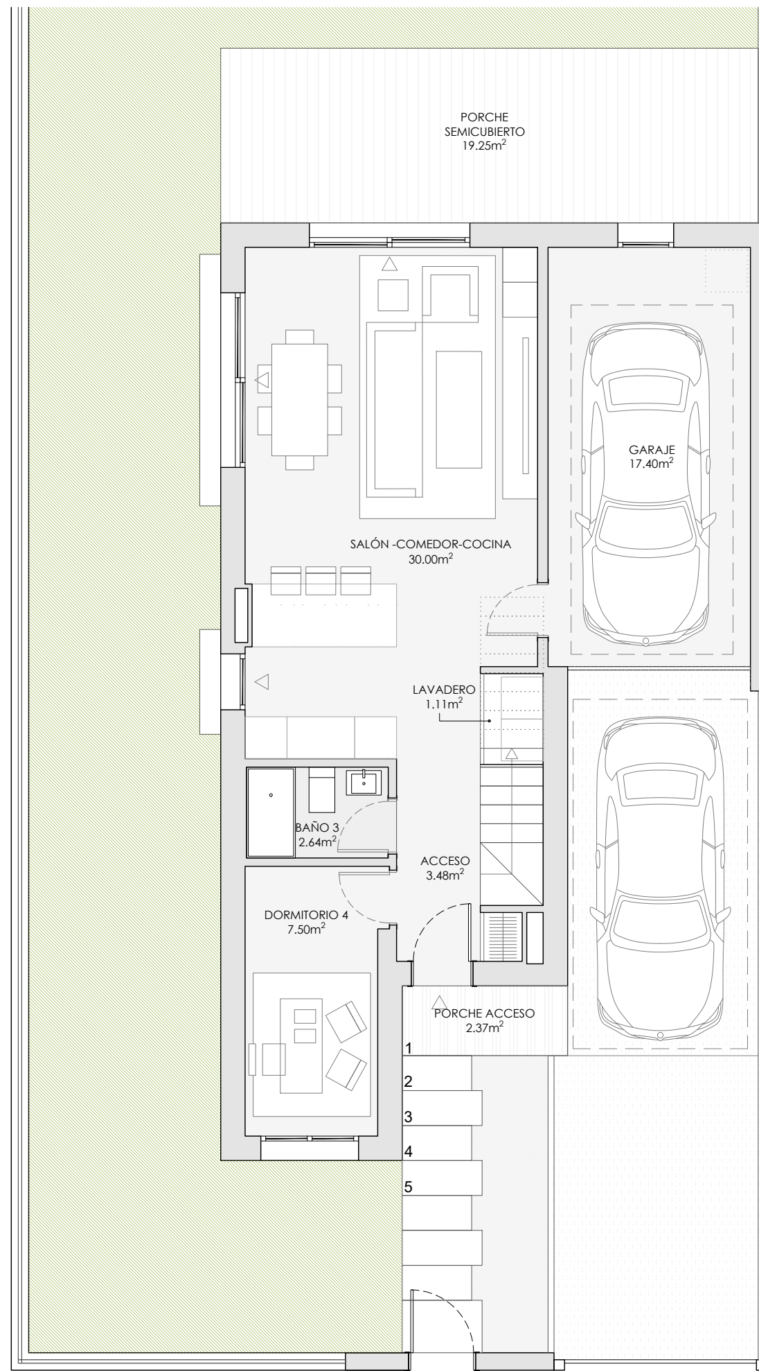
PLANTA BAJA
