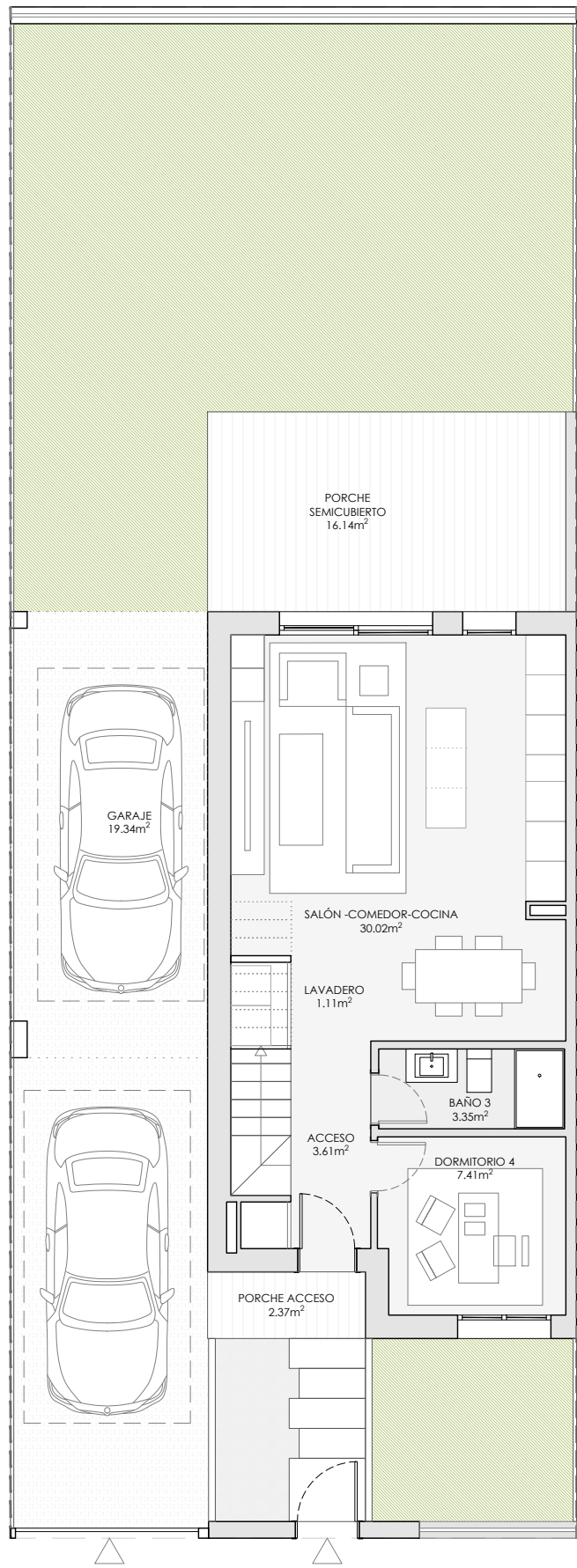
PLANTA BAJA
