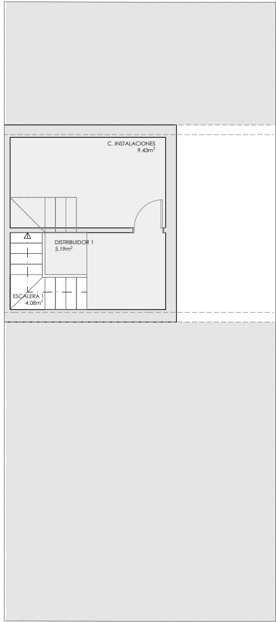
PLANTA SÓTANO
