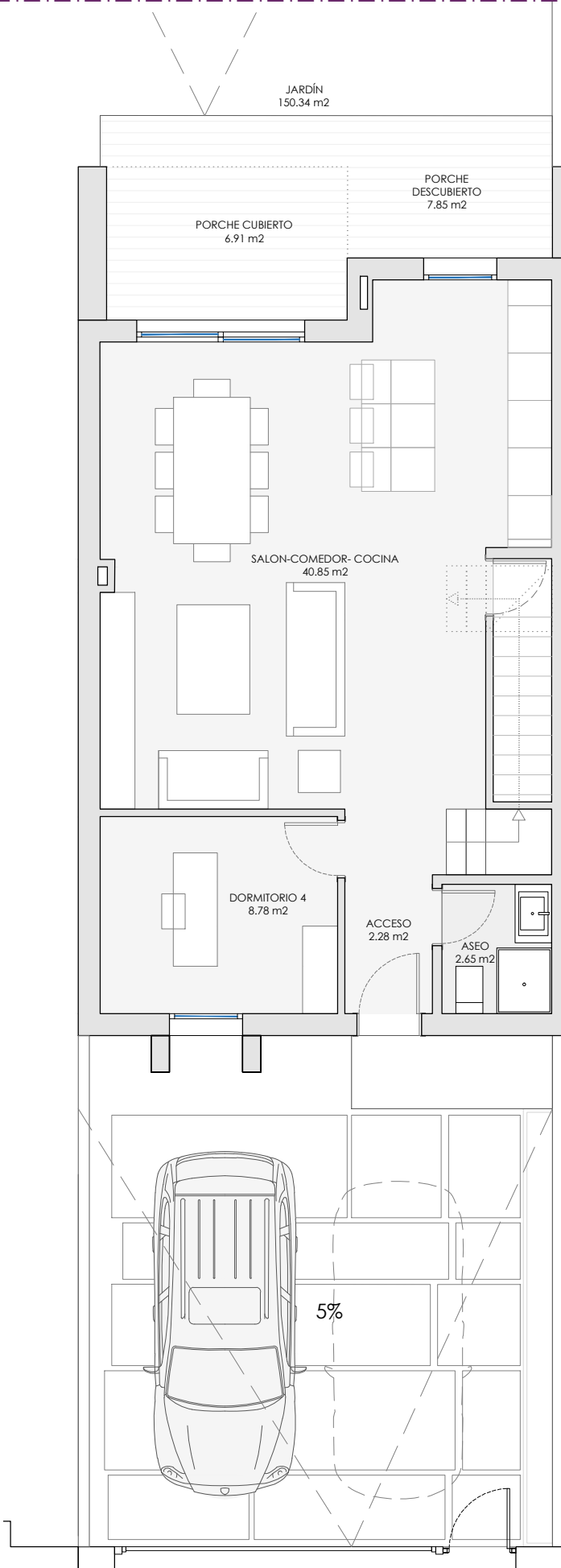
PLANTA BAJA
