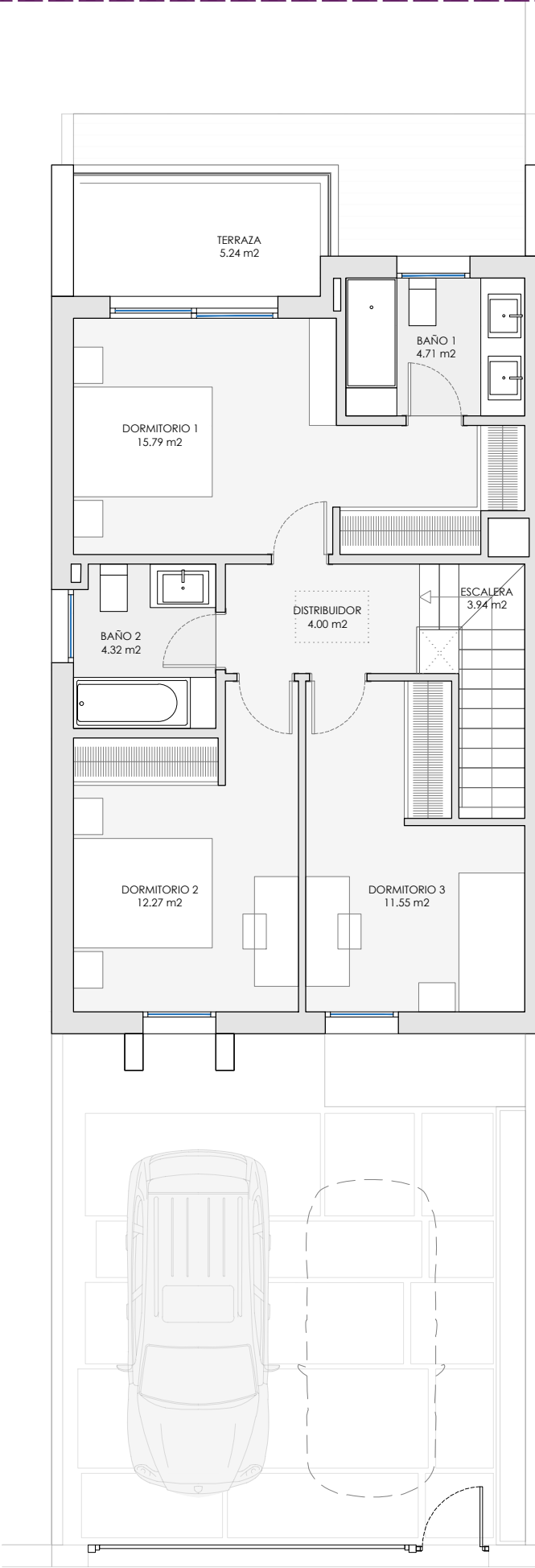
PLANTA PRIMERA
