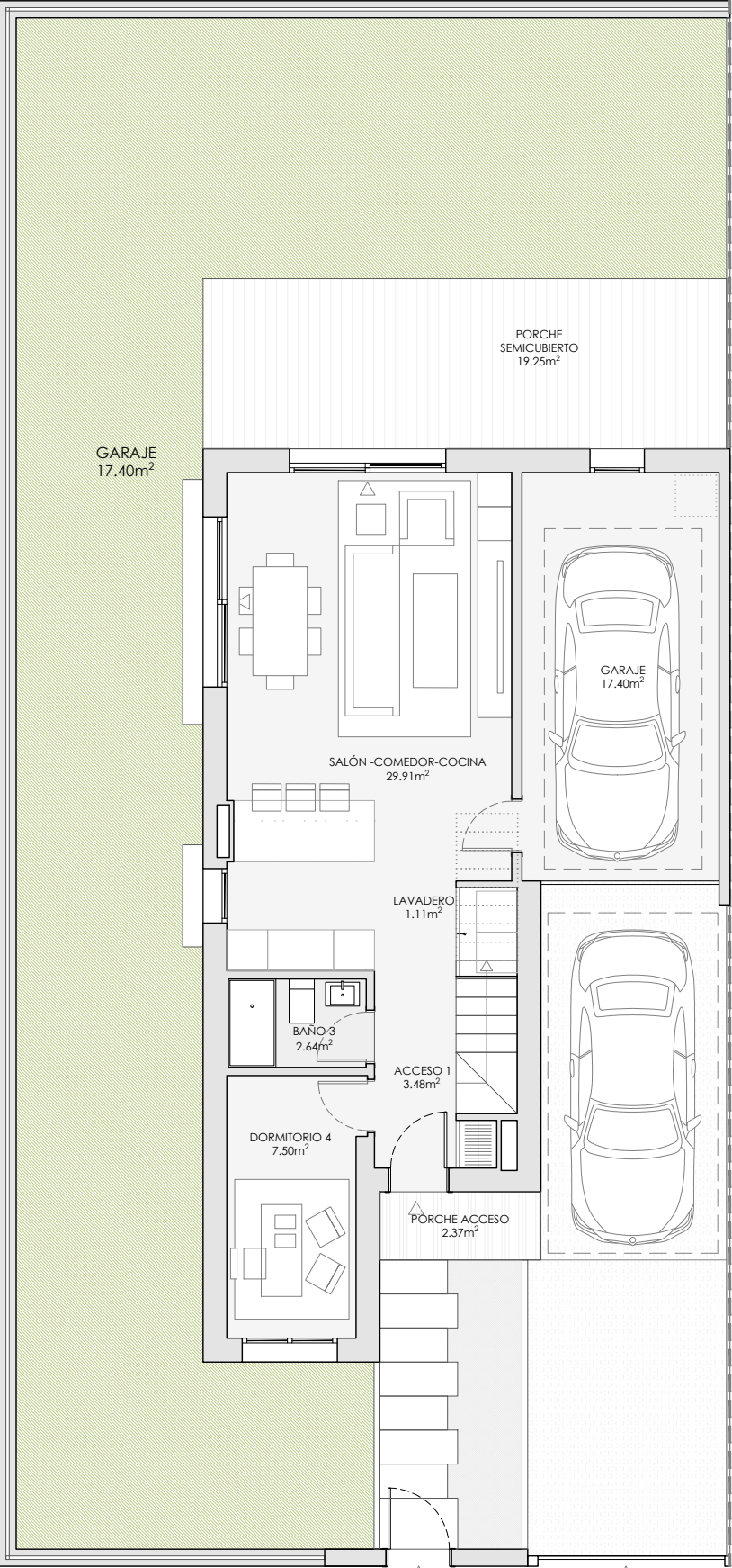
PLANTA BAJA
