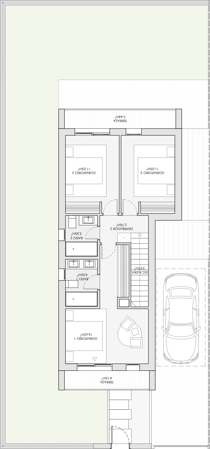
PLANTA PRIMERA
