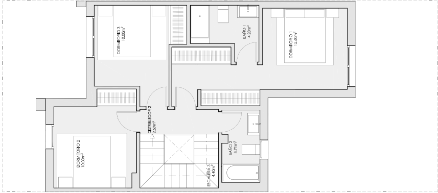
PLANTA PRIMERA
