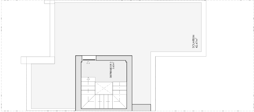
PLANTA CUBIERTA
