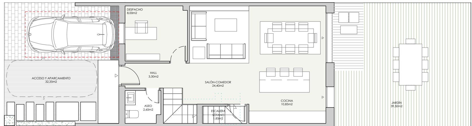
PLANTA BAJA
