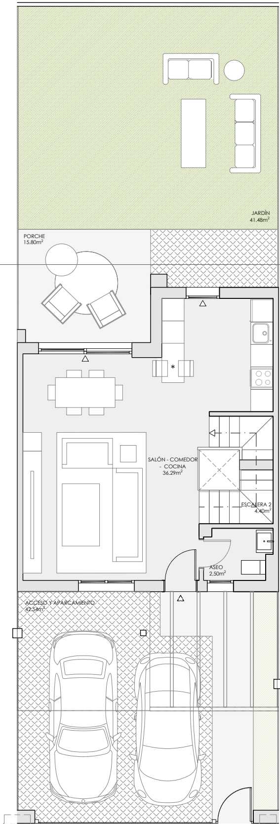
PLANTA BAJA
