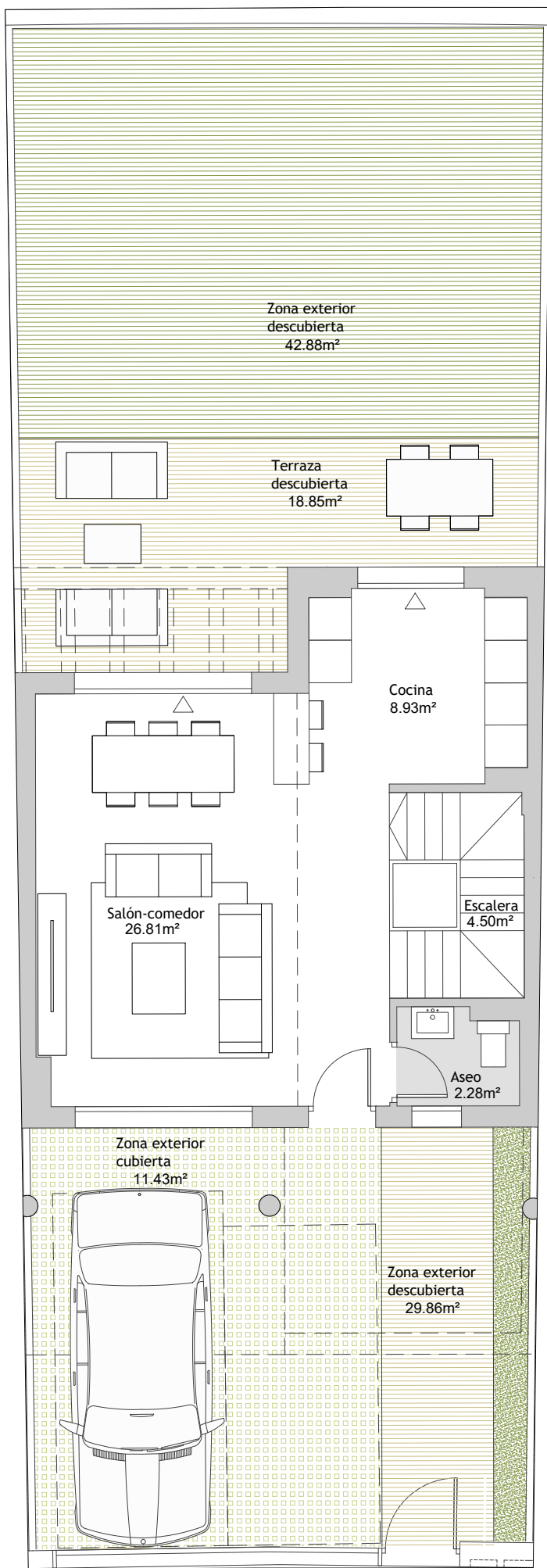
PLANTA BAJA
