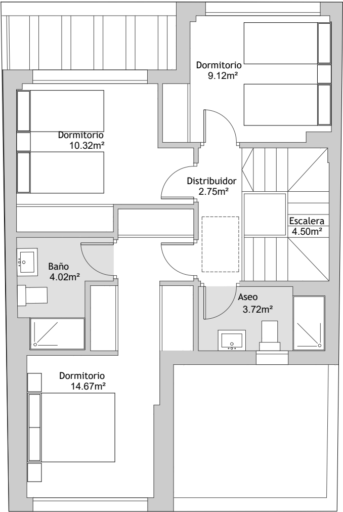
PLANTA PRIMERA
