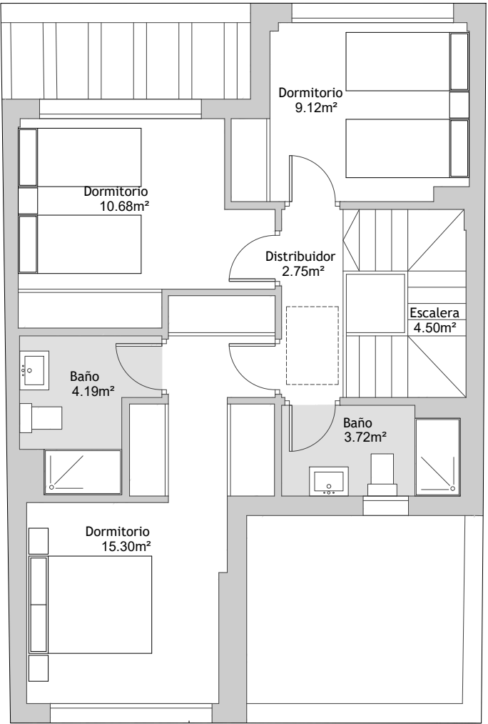
PLANTA PRIMERA
