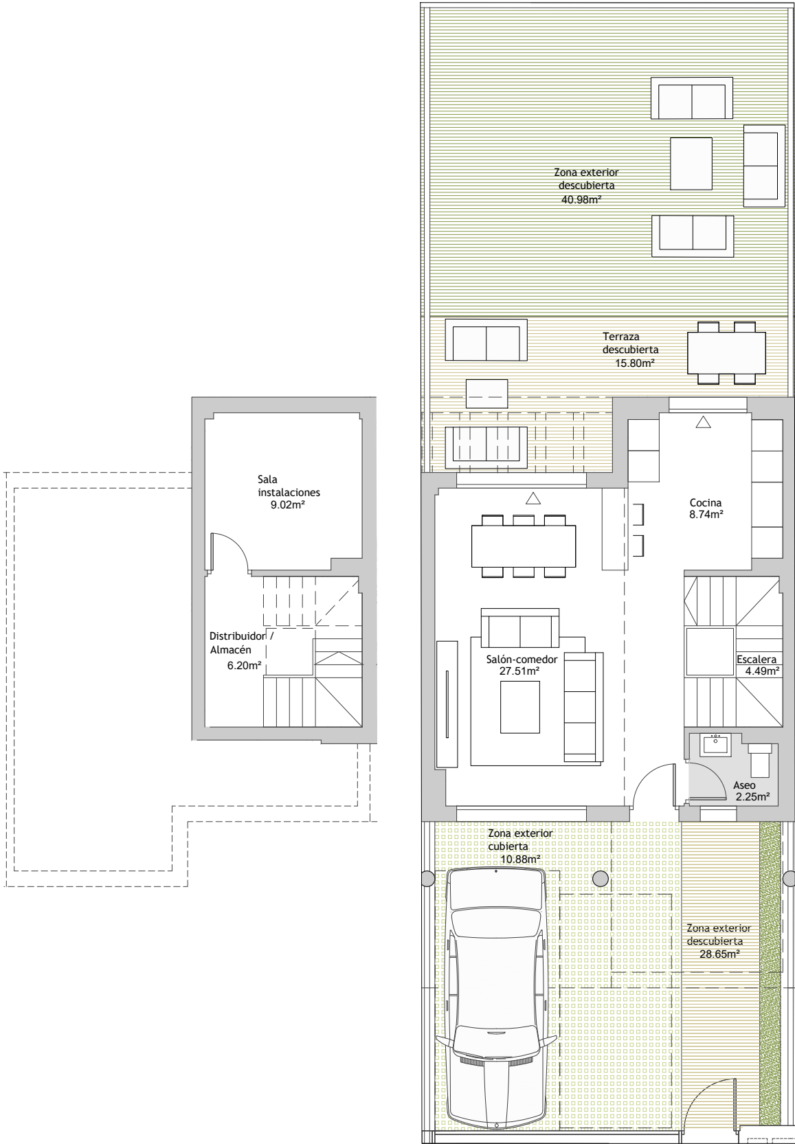
PLANTA SÓTANO
