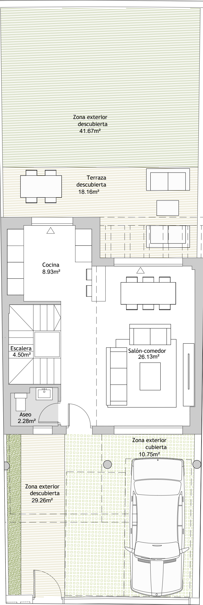
PLANTA BAJA
