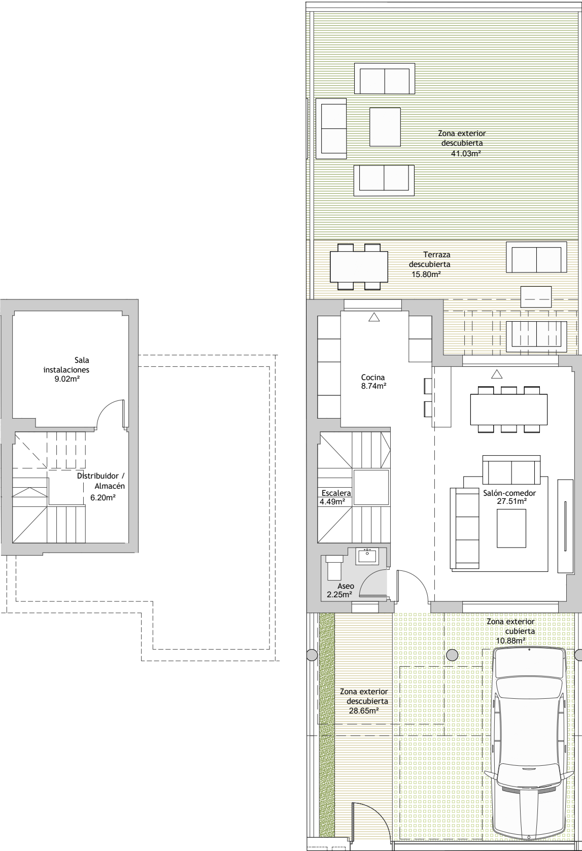
PLANTA SÓTANO
