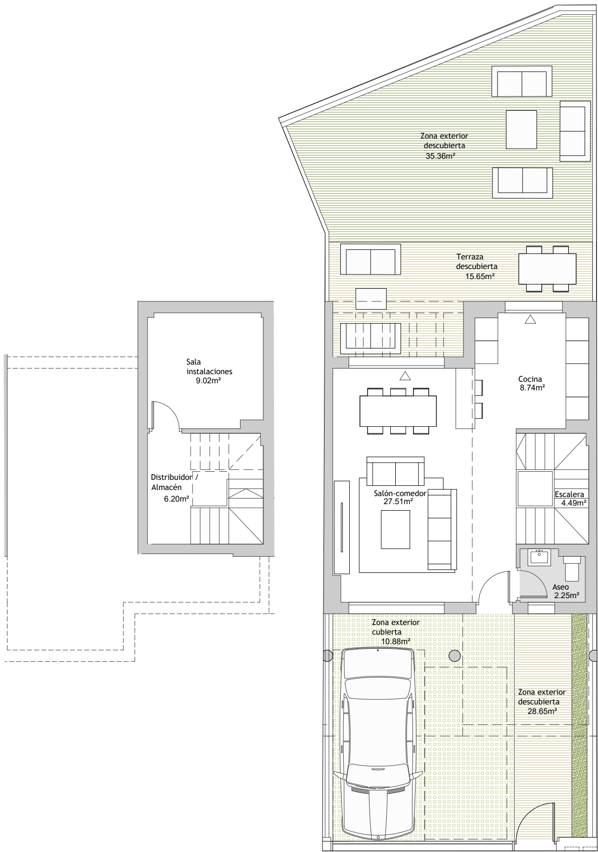
PLANTA SÓTANO
