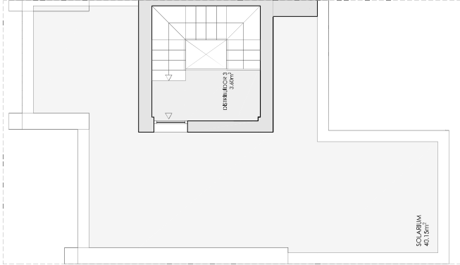
PLANTA CUBIERTA
